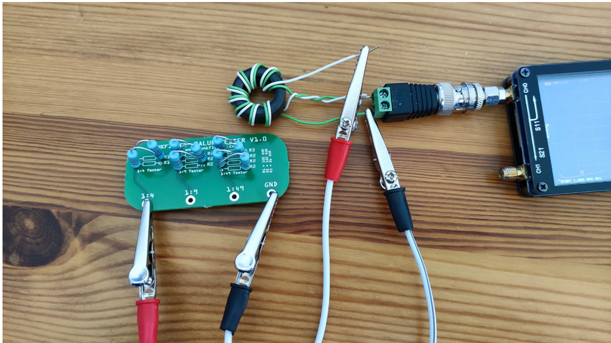
1:4 Balun oder UnUn
